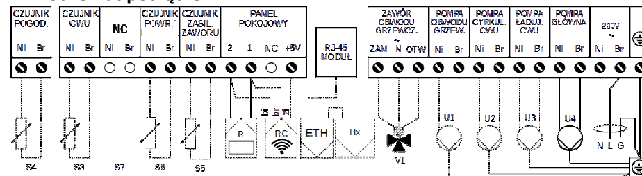
Schemat podłączeń:
