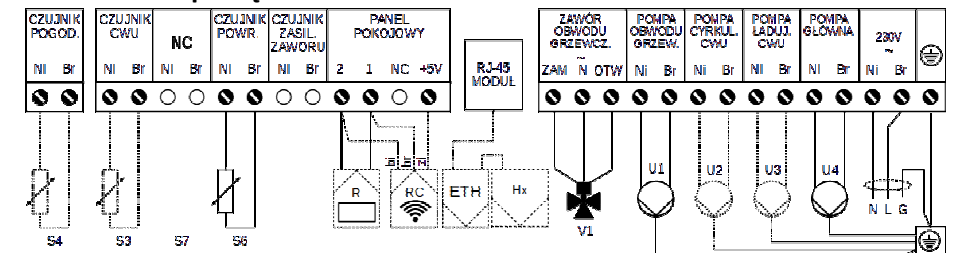
Schemat podłączeń:
