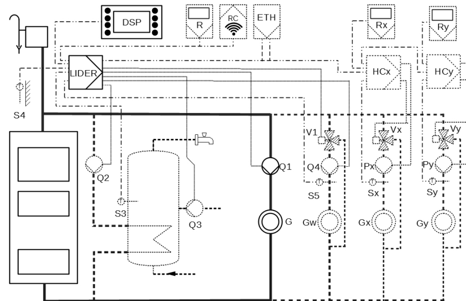
Schemat podłączeń:
