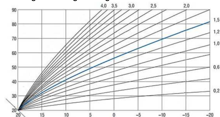
Rys. Krzywe grzewcze.
