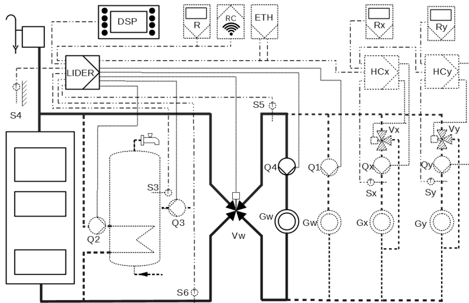
Schemat podłączeń:
