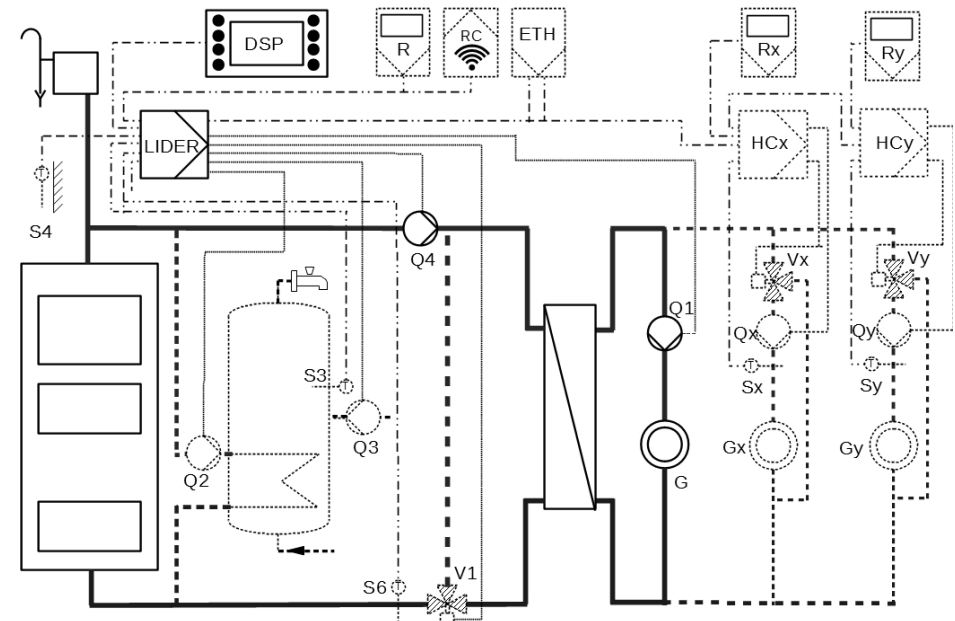
Schemat podłączeń:
